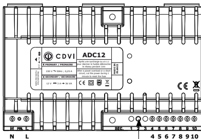
LED : Présence de tension de sortie
